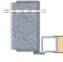
U - 60 x väggtj x 5 mm
